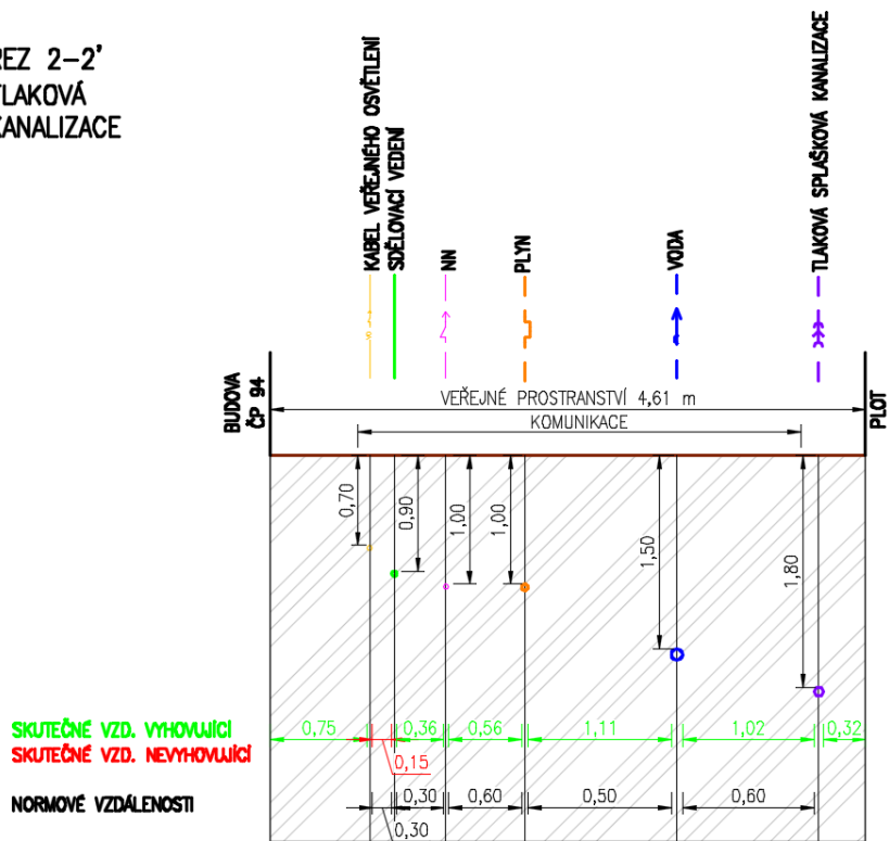
ŘEZ 2-2' GRAVITAČNÍ KANALIZACE
